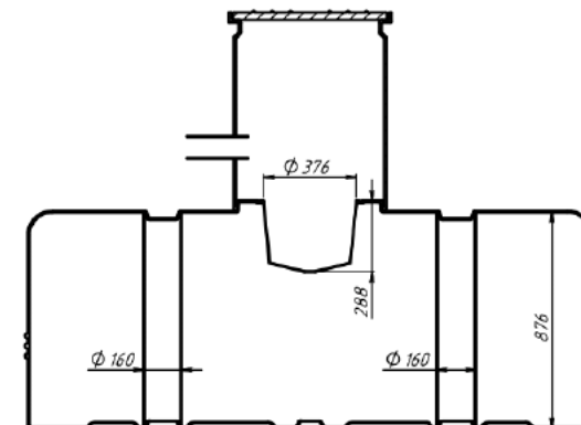
CROSS-SECTION A:A SCALE 1:12
