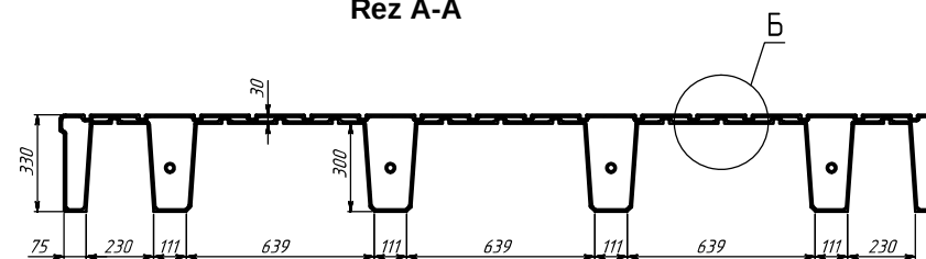
Řez A-A
