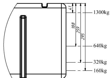
Závislost ponoru na zatížení
