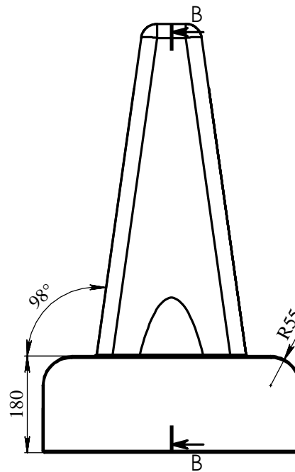
ŘEZ B-B MĚŘITKO 1:5
