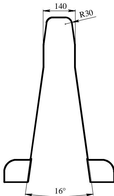
ŘEZ B-B MĚŘITKO 1:5
